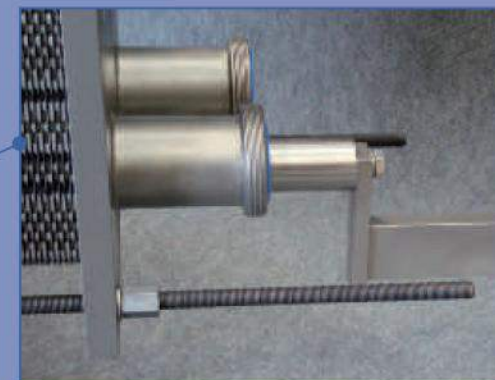
Barre inférieure avec décrochage pour montage aisé des plaques
